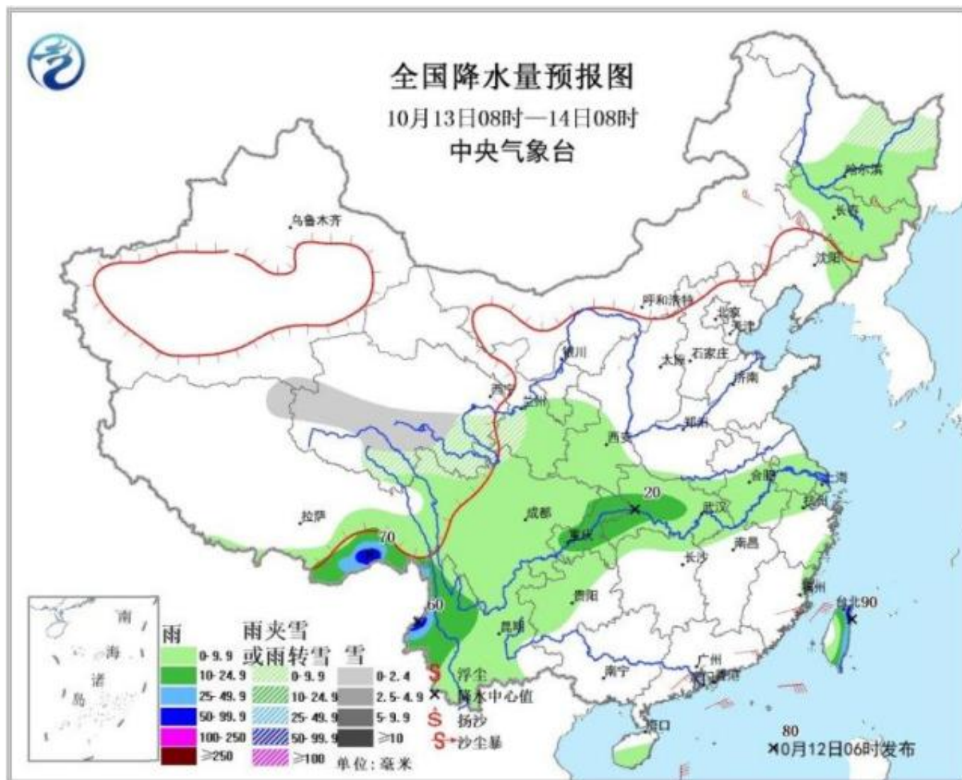
图2 全国降水量预报图(10月13日08时-14日08时)
